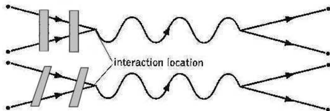
Figura 6.11 Dos observadores en movimiento relativo coinciden en dónde y cuándo interaccionan mutuamente dos partículas puntuales.
