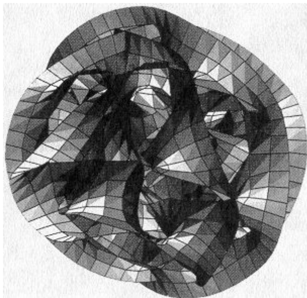
Figura 8.9 Ejemplo de espacio de Calabi-Yau.
