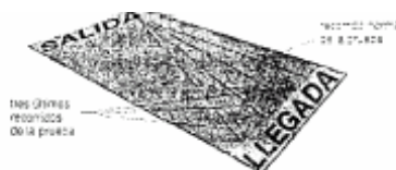
Figura 2.5 Debido al deslumbramiento producido por el sol al final de la tarde, Slim condujo con un ángulo de desviación cada vez mayor durante los tres últimos recorridos.
