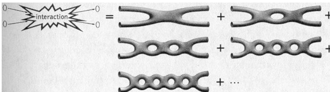
Figura 12.6 La influencia neta que cada cuerda que ingresa tiene sobre las otras viene de sumar todas las influencias que involucran diagramas con aún más bucles.
