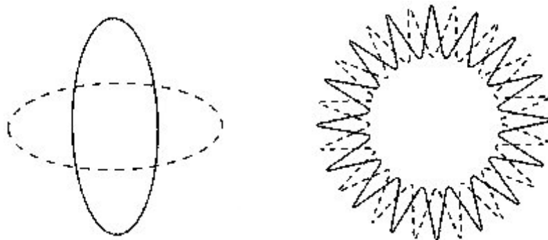
Figura 6.3 Los patrones vibratorios más frenéticos tienen más energía que los menos frenéticos.
