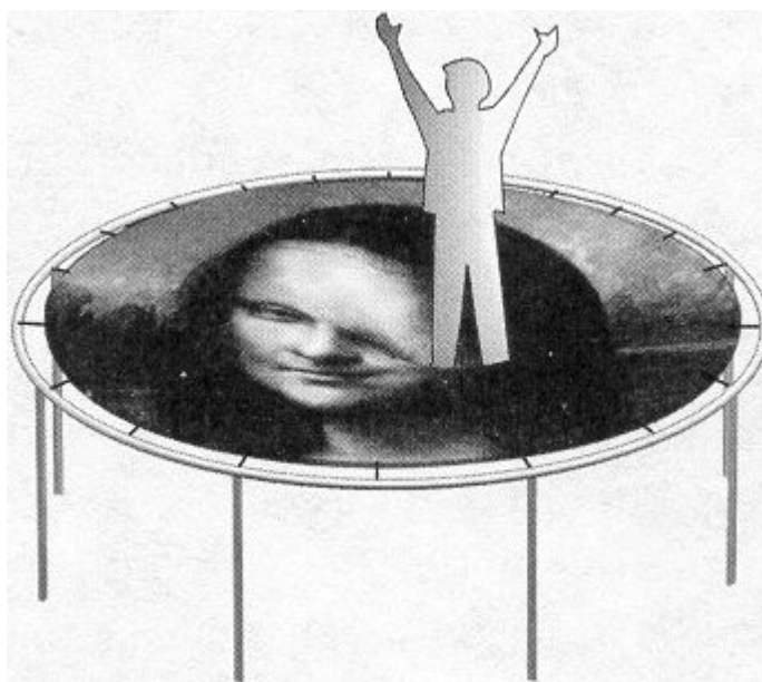
Figura 10.1 Si una persona se sitúa en pie sobre una cama elástica con la figura de la Mona Lisa, la imagen se distorsiona al máximo justo bajo los pies, debido al peso de dicha persona.
