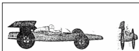
Figura 2.4 Un objeto en movimiento es acortado en la dirección de su movimiento.
