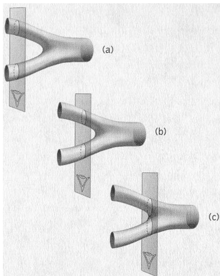
Figura 6.8 Las dos cuerdas entrantes vistas desde la perspectiva de George en tres momentos consecutivos en el tiempo. En (a) y (b) las cuerdas se acercan cada vez más la una a la otra, en (c) se tocan por primera vez, desde la perspectiva de George.
