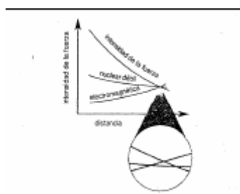
Figura 7.2 Un refinamiento en el cálculo de las intensidades de las fuerzas pone de manifiesto que sin la supersimetría casi llegan a coincidir, pero no lo hacen.
