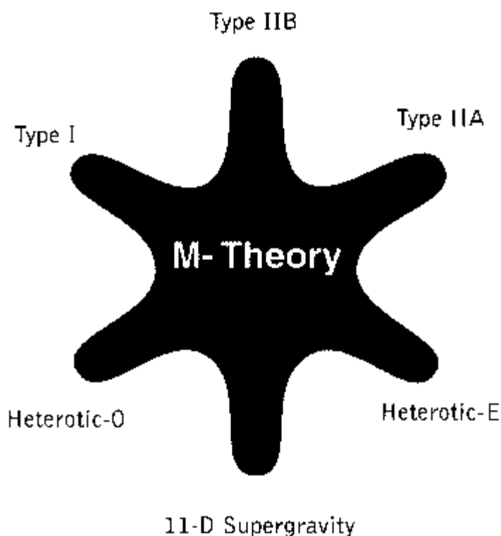
Figura 12.11 Incorporando las dualidades, las cinco teorías de cuerdas, la supergravedad de once dimensiones, y la Teoría-M se mezclan en un marco unificado.
