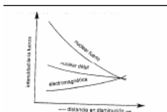
Figura 7.1 Las intensidades de las tres fuerzas no gravitatorias cuando operan a escalas de distancias cada vez más cortas o, lo que es equivalente, cuando actúan sobre procesos de energía cada vez mayor.
