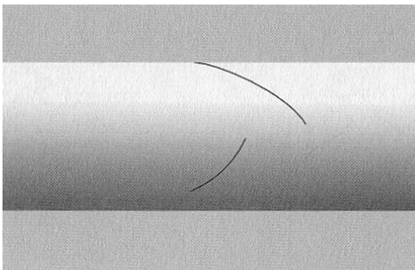
Figura 8.5 Un ser lineal puede ver directamente en el interior del cuerpo de otro cuando Linealandia se expande dentro del universo de la manguera.
