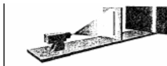
Figura 4.4 La rendija derecha está abierta en este experimento, provocando una imagen sobre la placa fotográfica como la que se muestra.
