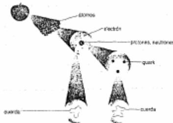
Figura 1.1 La materia está compuesta por átomos, que a su vez están hechos de quarks y electrones. Según la teoría de cuerdas, todas estas partículas son en realidad diminutos bucles de cuerda vibrante.
