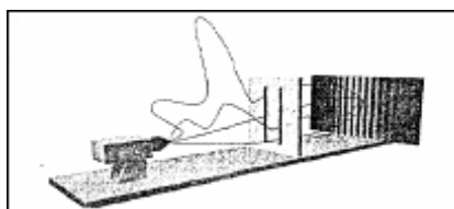
Figura 4.10 Según la formulación de Feynman de la mecánica cuántica, se debe considerar que las partículas se desplazan de un lugar a otro recorriendo todas las trayectorias posibles. Aquí se muestran unas pocas de las infinitas trayectorias de un único electrón que se desplaza desde la fuente de emisión hasta la pantalla fosforescente. Obsérvese que este único electrón atraviesa en realidad ambas rendijas.
