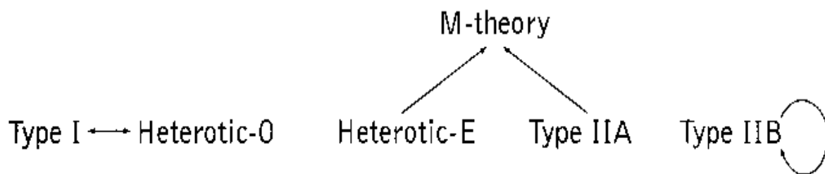
Figura 12.9 Las flechas muestran cuales teorías son duales con otras.
