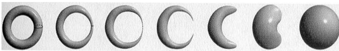
Figura 13.3 Un pedazo circular de una rosquilla (un toro) se colapsa en un punto. La superficie se abre rasgándose, produciendo dos agujeros puntuales. Una esfera de cero dimensiones (dos puntos) se "pega", reemplazando la esfera original unidimensional (el círculo) y reparando la superficie rasgada. Esto permite la transformación a una forma completamente diferente —una pelota de playa—.
