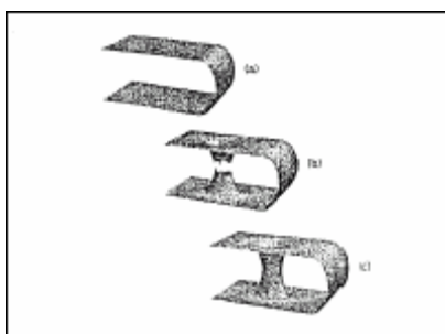
Figura 11.1 (a) En un universo con «forma de U», el único modo de ir de un extremo al otro es atravesando todo el cosmos. (b) La estructura del espacio se raja, y los dos extremos del wormhole empiezan a crecer. (c) Los dos extremos del wormhole se conectan, formando un nuevo puente — un atajo— desde un extremo del universo hasta el otro.
