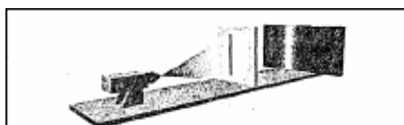
Figura 4.5 Como en la Figura 4.4, salvo que ahora es la rendija de la izquierda la que está abierta.
