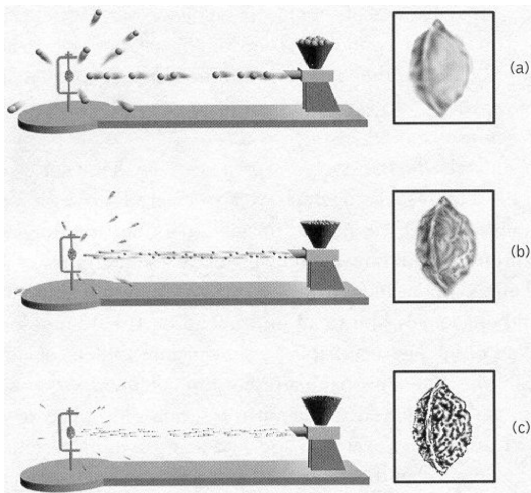
Figura 6.4 Un hueso de melocotón se fija en un tornillo de banco y se dibuja exclusivamente observando cómo se desvían los objetos «sondas» lanzados contra dicho hueso. Utilizando sondas aún más pequeñas -(a) canicas, (b) perdigones de cinco milímetros, (c) perdigones de medio milímetro- se pueden dibujar imágenes aún más detalladas.
