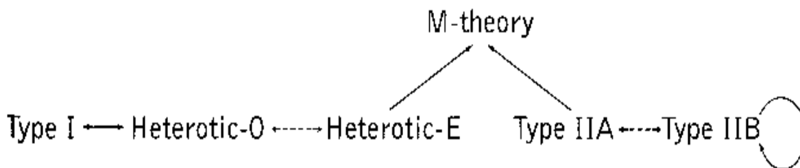
Figura 12.10 Incluyendo las dualidades que involucran la forma geométrica del espacio-tiempo (como en el Capítulo 10), las cinco teorías de cuerdas y la Teoría-M se reúnen en una red de dualidades.
