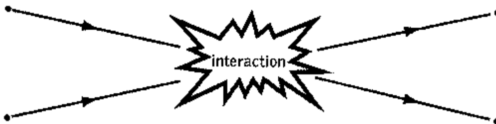
Figura 6.5 Dos partículas interactúan «chocan entre sí»— lo cual hace que la trayectoria de cada una de ellas sufra una desviación.
