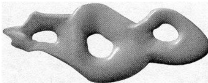
Figura 9.2 La forma de una rosquilla de múltiples asas se puede deformar de muchas maneras, una de las cuales se representa aquí, sin cambiar el número de agujeros que contiene.
