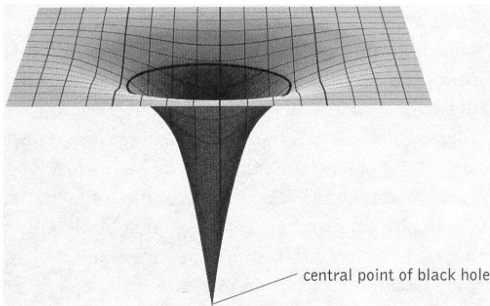
Figura 3.7 Un agujero negro hace que la estructura del espacio-tiempo que lo rodea se curve de una manera tan pronunciada que cualquier objeto que entra en el «horizonte de sucesos» - representado mediante el círculo oscuro- no puede escapar de su atracción gravitatoria. Nadie sabe exactamente qué es lo que sucede en el punto más profundo del interior de un agujero negro.
