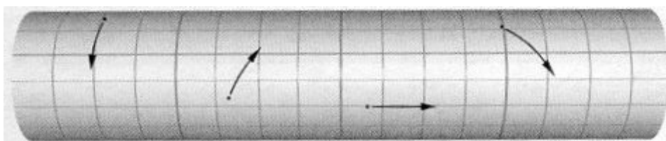
Figura 10.2 Partículas puntuales moviéndose sobre un cilindro.
