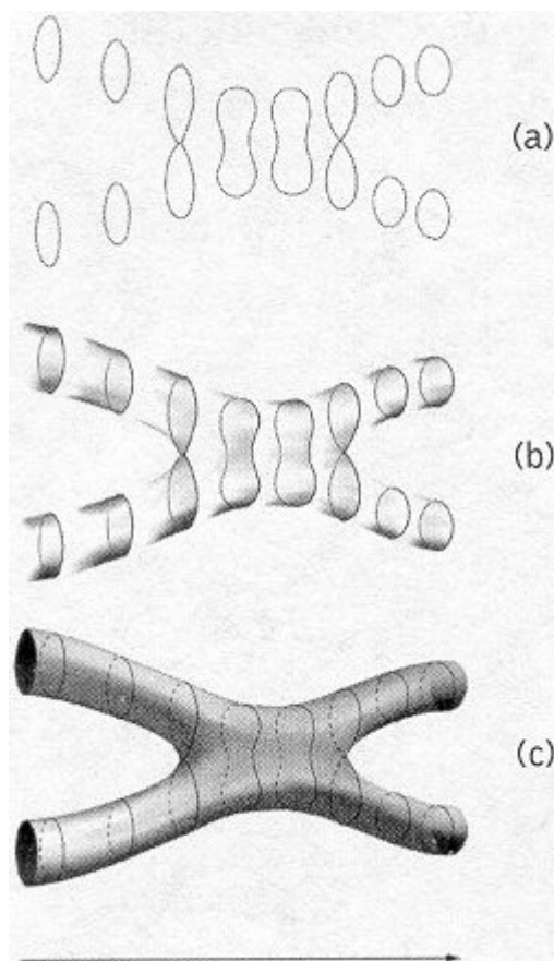
Figura 6.7 (a) Dos cuerdas, en un proceso de colisión, pueden unirse para dar lugar a una tercera cuerda, que posteriormente puede escindir en dos cuerdas que se desplazan siguiendo trayectorias desviadas (b). El mismo proceso que se representa en (a), enfatizando el movimiento de las cuerdas (c). Una «fotografía de lapso de tiempo» en la que las dos cuerdas que interaccionan barren una «lámina universal».
