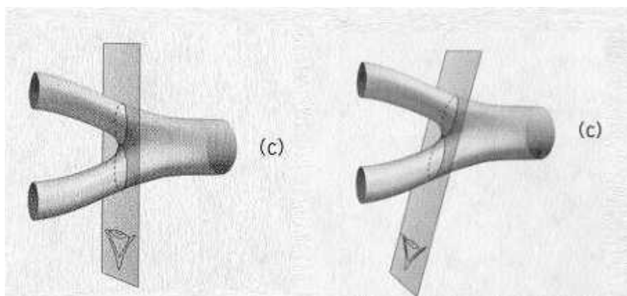
Figura 6.10 George y Gracie no están de acuerdo sobre la posición de la interacción.
