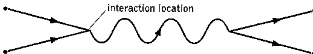
Figura 6.6 En la teoría de campos cuántica, una partícula y su antipartícula pueden momentáneamente aniquilarse mutuamente, produciendo un fotón. Luego, este fotón puede originar otra partícula y antipartícula que viajan en diferentes trayectorias.
