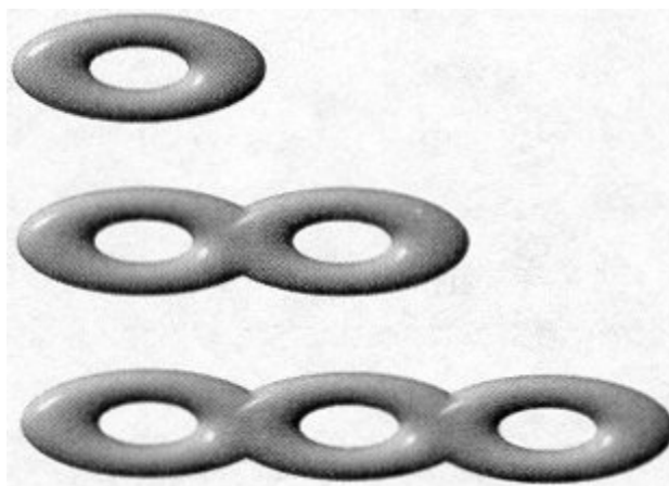
Figura 9.1 Una rosquilla, o toro, y sus primos de varias asas.
