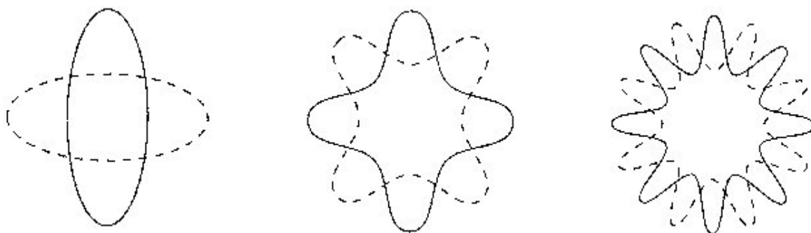
Figura 6.2 En la teoría de cuerdas, los bucles pueden vibrar mediante patrones de resonancia -similares a los de las cuerdas del violín- en los que un número entero de picos y senos encaja a lo largo de su extensión espacial.
