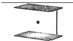
Figura 2.1 Un reloj de luz consiste en dos espejos paralelos y un fotón que salta rebotando sobre dichos espejos. El reloj hace «tic» cada vez que el fotón realiza un viaje completo de ida y vuelta.
