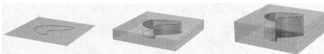
Figura 12.7 A medida que se incrementa la constante de acoplamiento de la cuerda Heterótica-E, una nueva dimensión espacial aparece y la cuerda misma se estira hasta adoptar una forma de membrana cilíndrica.
